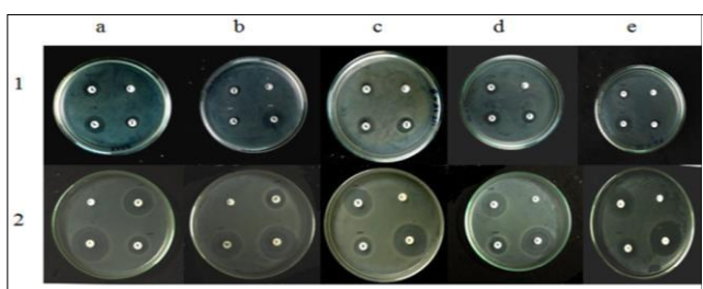
Fig 3: Antibacterial activity 1) A. tenuissima 2) C. gloeosporioides . a) E. coli b) K. pneumonia c) B. subtilis d) S. typhi e) S. aureus . C- Negative control, A – Ampicillin, S – Streptomycin, T- Test
